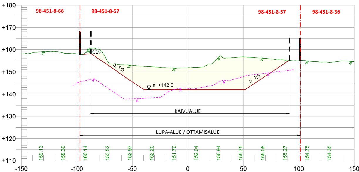
POIKKILEIKKAUS 400-400 1:2000 / 1:1000
