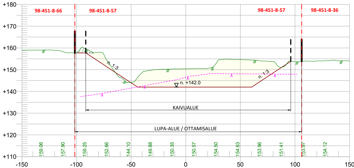
POIKKILEIKKAUS 300-300 1:2000 / 1:1000
