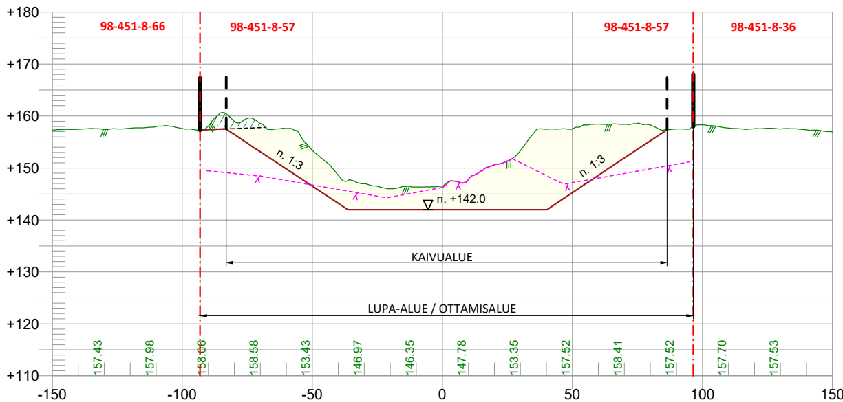
POIKKILEIKKAUS 500-500 1:2000 / 1:1000
