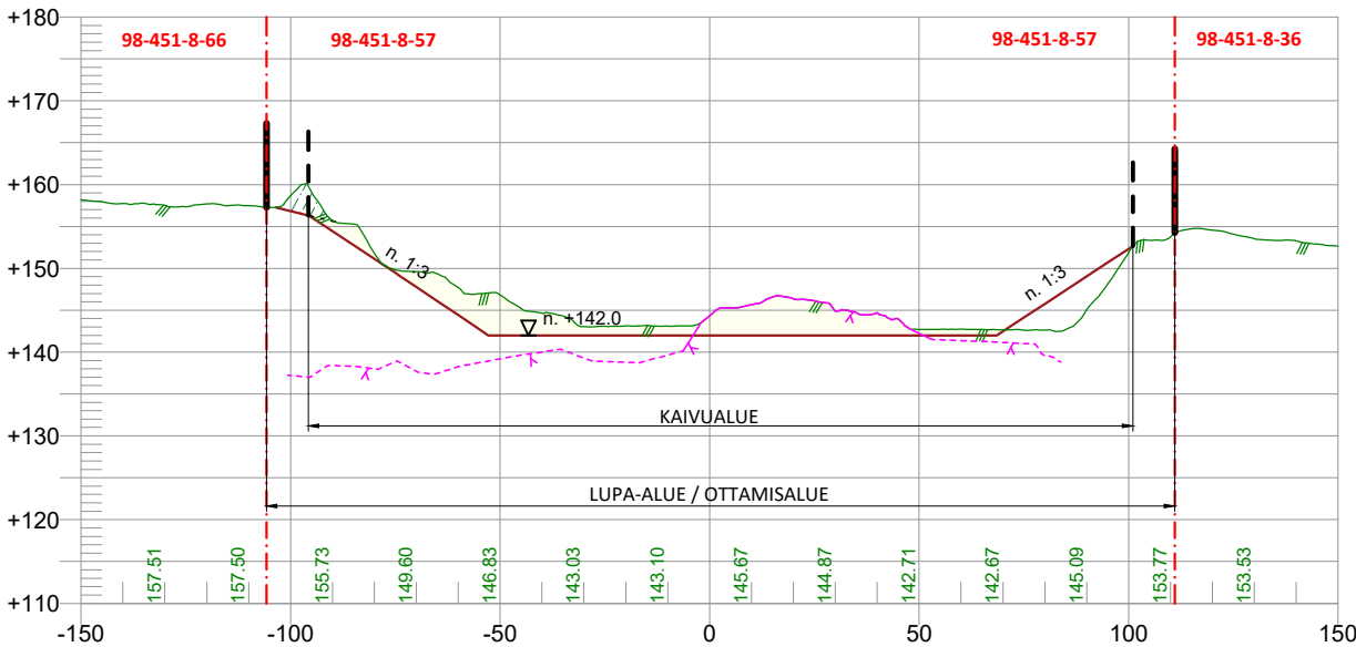
POIKKILEIKKAUS 200-200 1:2000 / 1:1000
